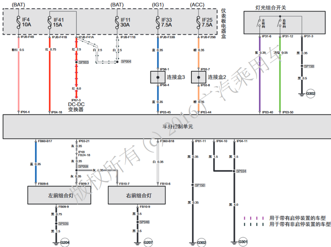
26-1 转向灯和危急警告灯电路图
